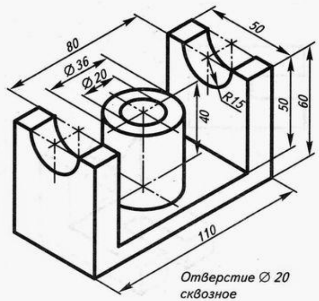
Стойка. Сталь
