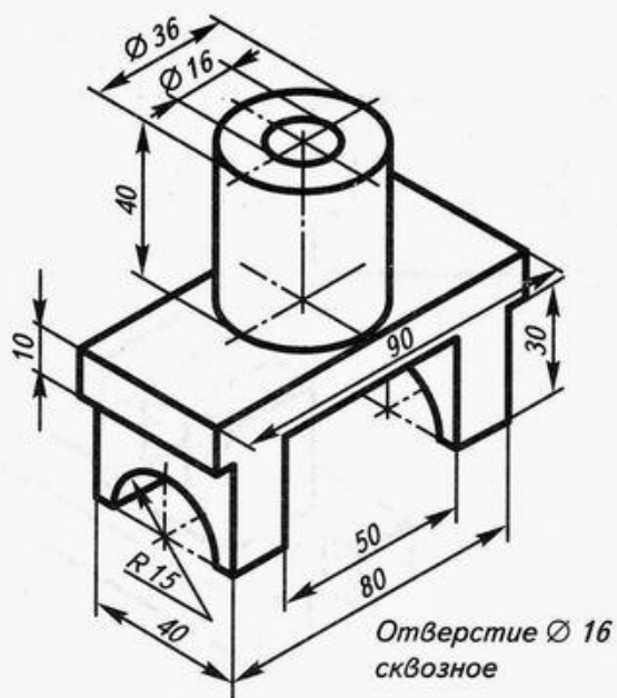
Ползун. Сталь
