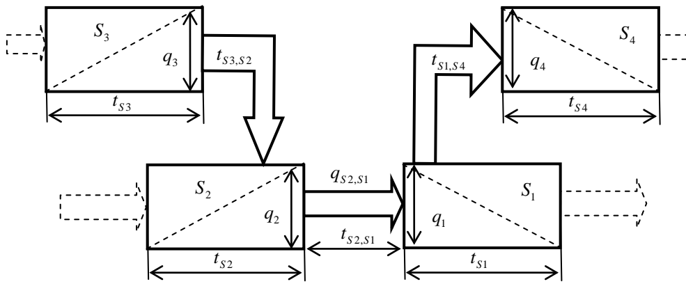
Рисунок 6 – Схема изменения структуры потоков в ПТК
