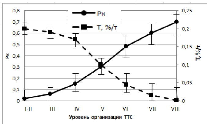
Рисунок 3 – Зависимость транспортных затрат и качества грузовых перевозок от уровня организации ТТС
