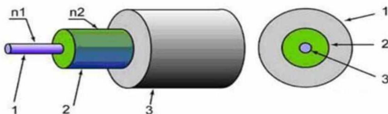
Рисунок 4 – Структура оптоволоконного кабеля:
